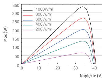
Krzywa moc-napięcie JAM60S10-335/MR-BF
