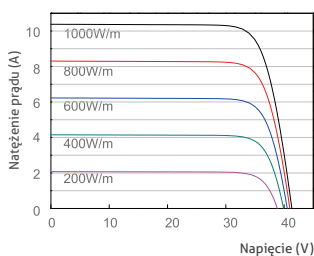
Krzywa prąd-napięcie JAM60S10-335/MR-BF
