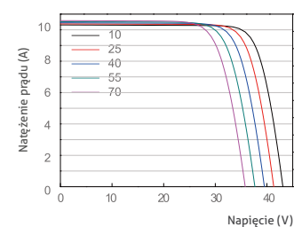
Krzywa prąd-napięcie JAM60S10-335/MR-BF
