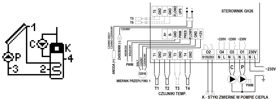
Schemat 5. Schemat ideowy oraz elektryczny instalacji nr 5.
