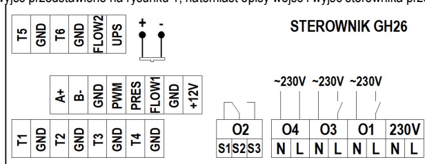
Rys. 1. Oznaczenia wejść i wyjść sterownika.
