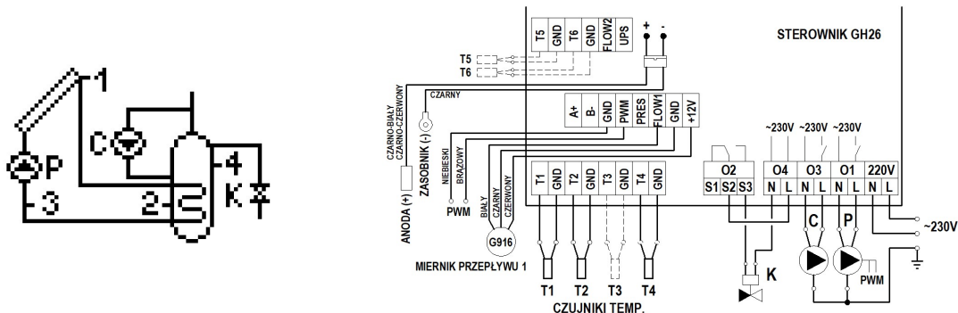
Schemat 17. Schemat ideowy oraz elektryczny instalacji układu nr 17.
