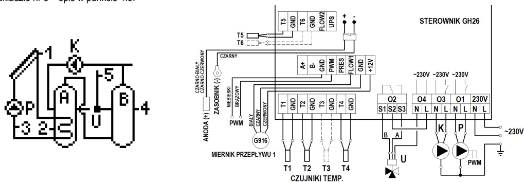
Schemat 19. Schemat ideowy oraz elektryczny instalacji układu nr 19.
