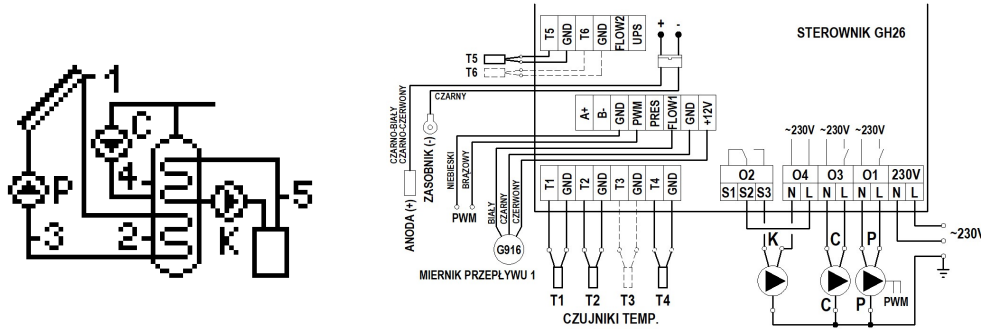
Schemat 6. Schemat ideowy oraz elektryczny instalacji nr 6.
