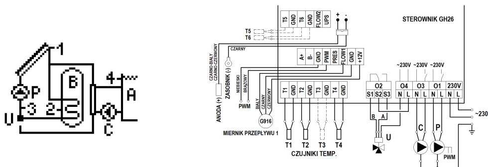
Schemat 9. Schemat ideowy oraz elektryczny instalacji nr 9.
