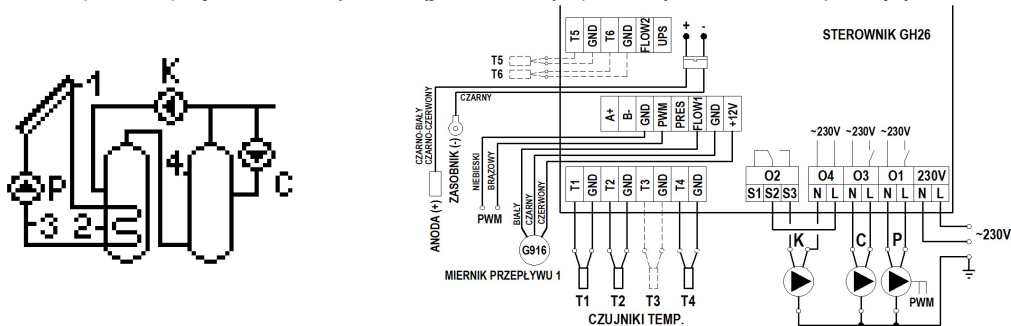
Schemat 7. Schemat ideowy oraz elektryczny instalacji nr 7.
