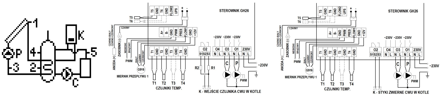
Schemat 14. Schemat ideowy oraz elektryczny instalacji układu nr 14.
