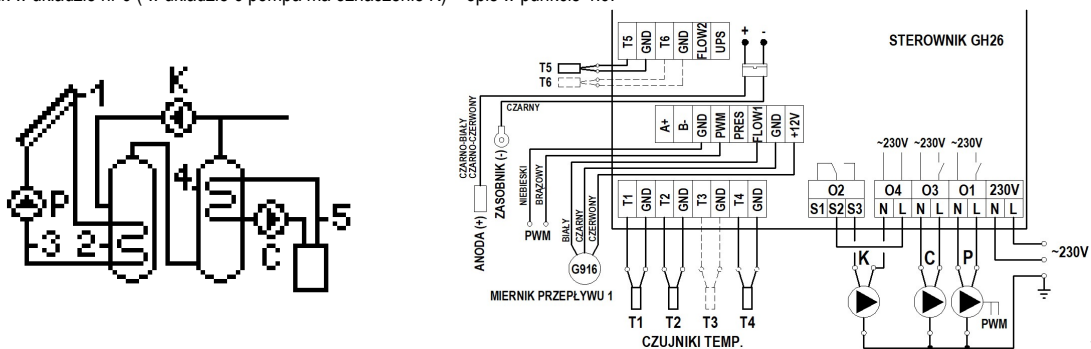
Schemat 18. Schemat ideowy oraz elektryczny instalacji układu nr 18.
