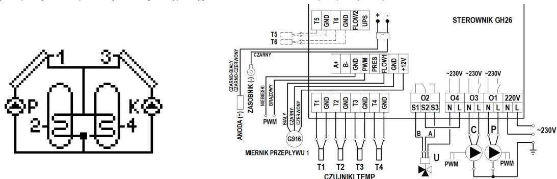
Schemat 16. Schemat ideowy oraz elektryczny instalacji układu nr 16.
