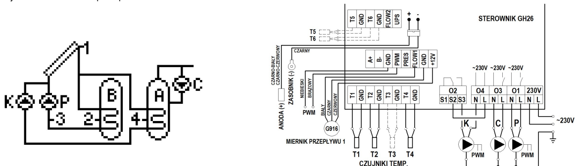
Schemat 12. Schemat ideowy oraz elektryczny instalacji układu nr 12.
