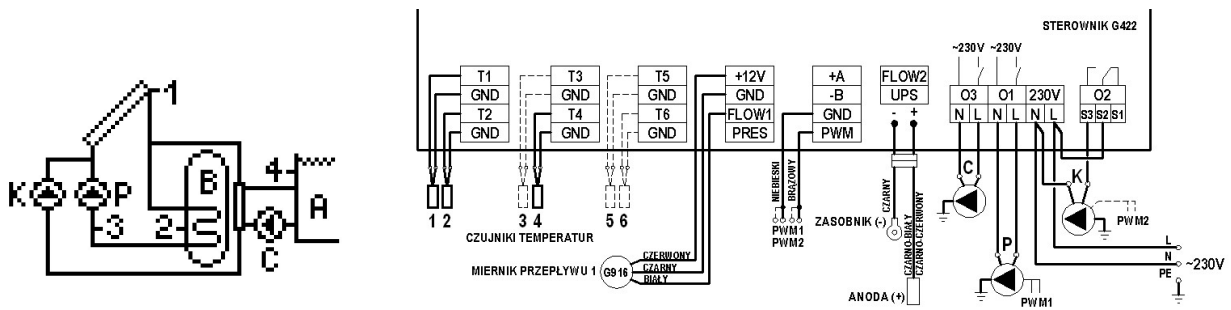
Schemat 10. Schemat ideowy oraz elektryczny instalacji nr 10.
