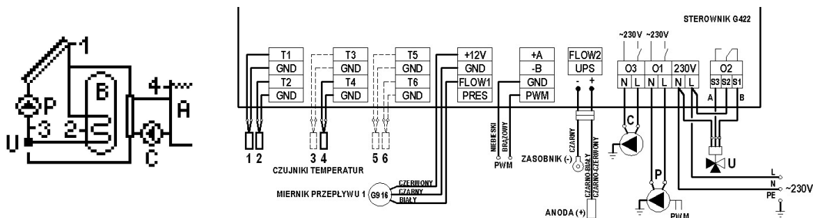
Schemat 9. Schemat ideowy oraz elektryczny instalacji nr 9.
