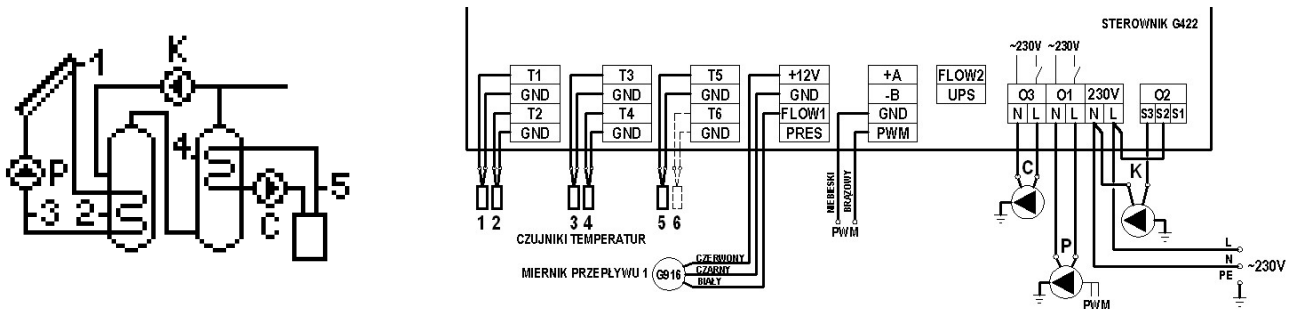
Schemat 18. Schemat ideowy oraz elektryczny instalacji układu nr 18.
