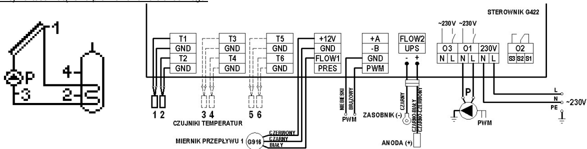
Schemat 1. Schemat ideowy oraz elektryczny instalacji nr 1.
