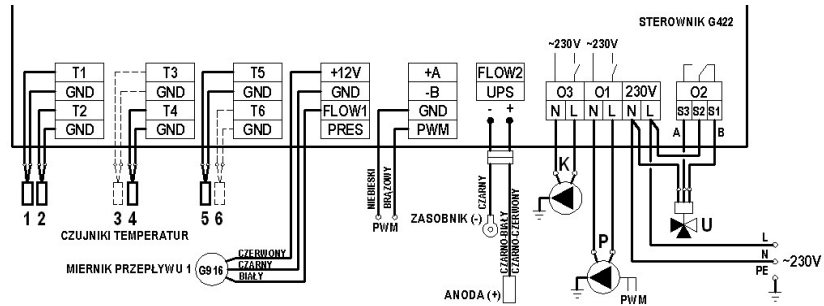
Schemat 19. Schemat ideowy oraz elektryczny instalacji układu nr 19.
