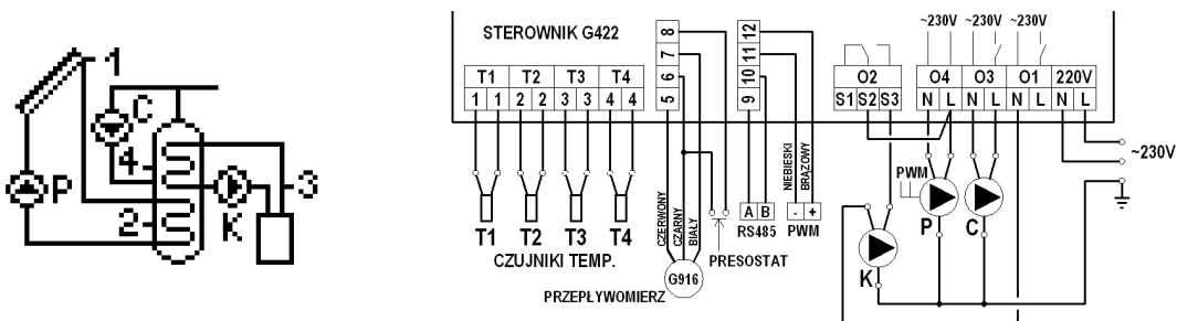
Schemat 6. Schemat ideowy oraz elektryczny instalacji nr 6.
