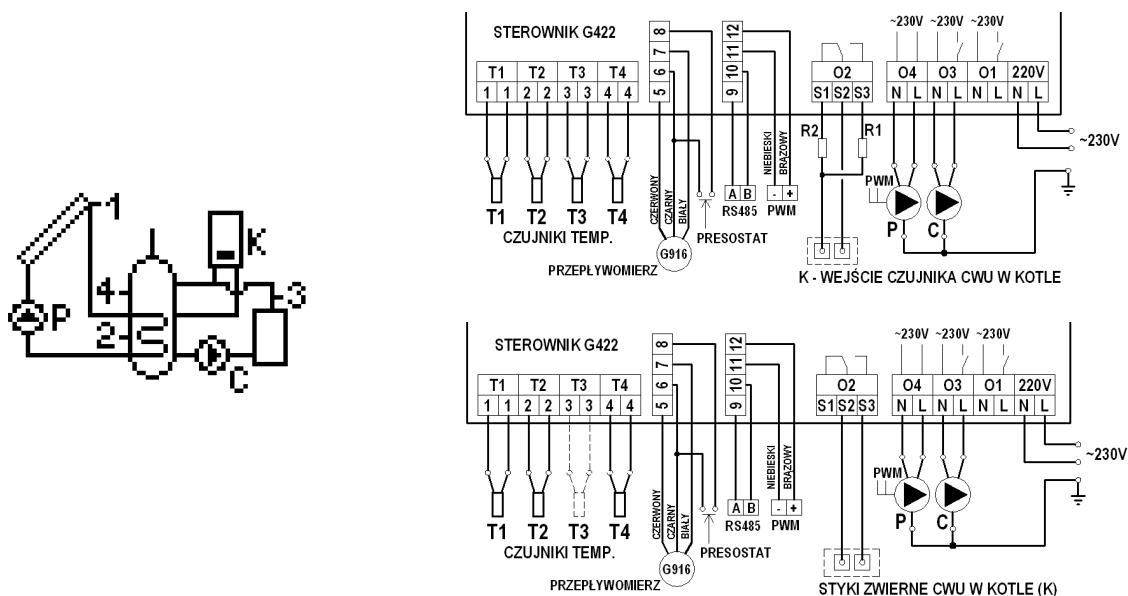
Schemat 14. Schemat ideowy oraz elektryczny instalacji układu nr 14.
