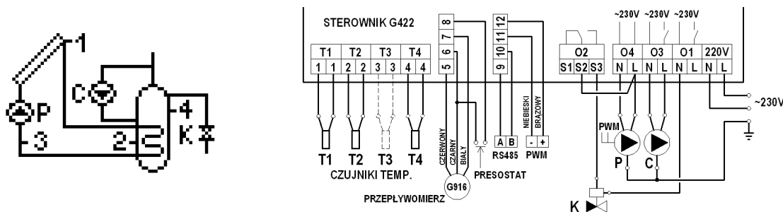
Schemat 17. Schemat ideowy oraz elektryczny instalacji układu nr 17.
