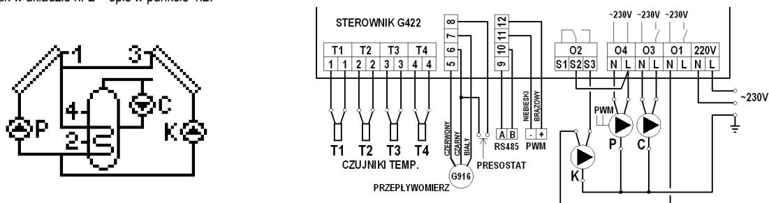
Schemat 15. Schemat ideowy oraz elektryczny instalacji układu nr 15.
