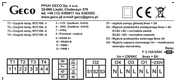
Rys. 1. Oznaczenie wejść i wyjść sterownika.
