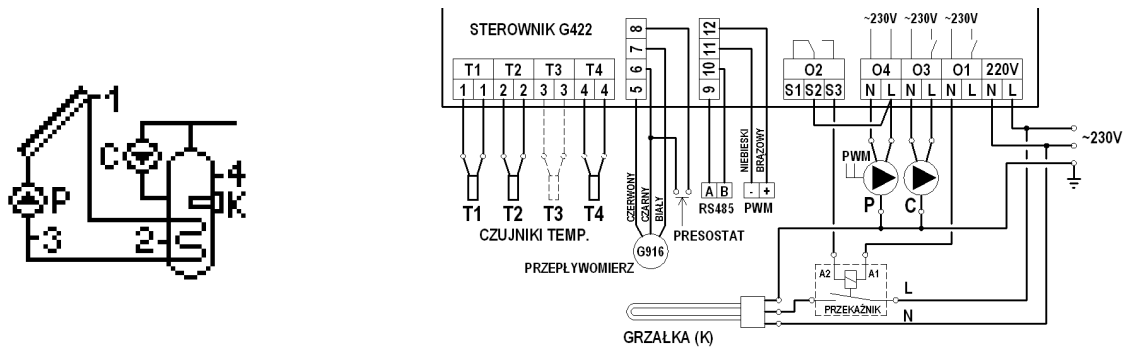
Schemat 4. Schemat ideowy oraz elektryczny instalacji nr 4.
