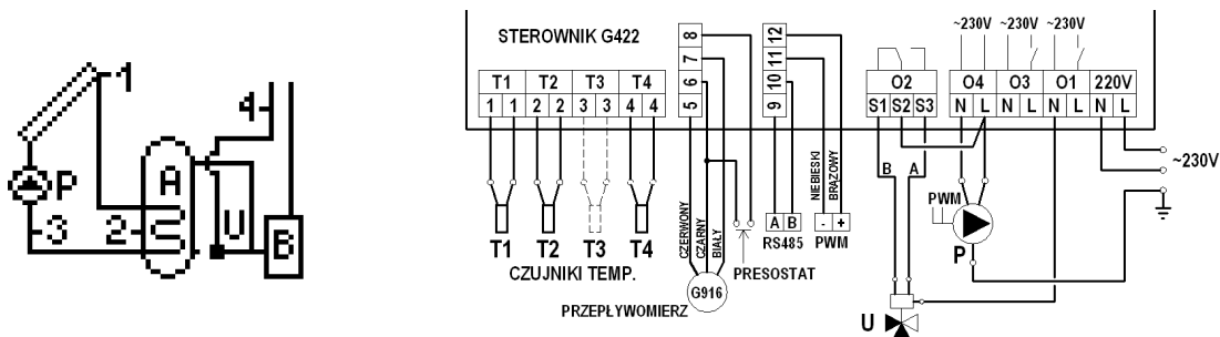
Schemat 13. Schemat ideowy oraz elektryczny instalacji układu nr 13.
