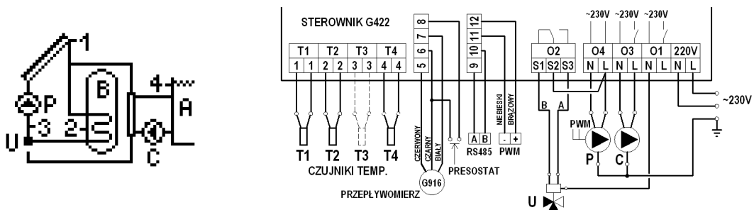
Schemat 9. Schemat ideowy oraz elektryczny instalacji nr 9.
