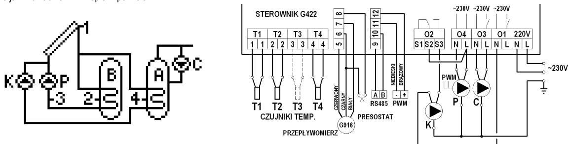
Schemat 12. Schemat ideowy oraz elektryczny instalacji układu nr 12.
