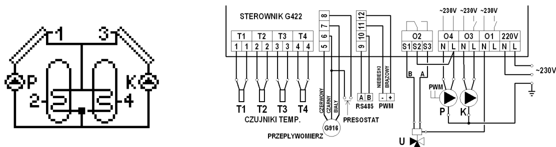
Schemat 16. Schemat ideowy oraz elektryczny instalacji układu nr 16.
