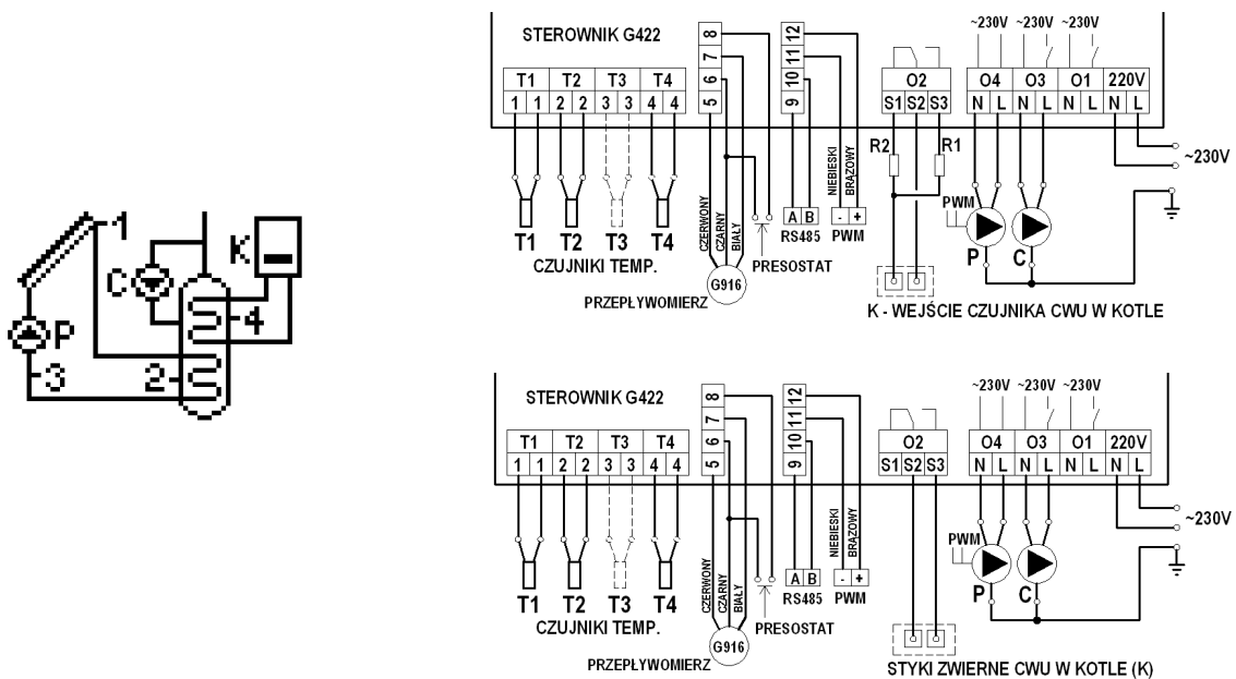
Schemat 3. Schemat ideowy oraz elektryczny instalacji nr 3.
