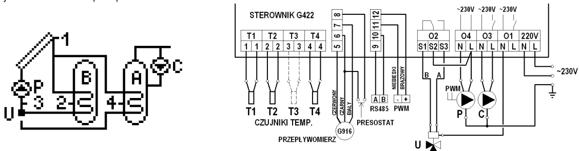
Schemat 11. Schemat ideowy oraz elektryczny instalacji układu nr 11.
