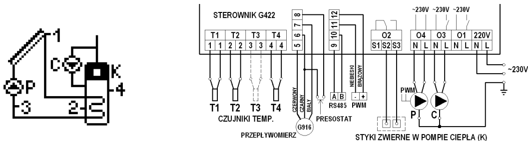
Schemat 5. Schemat ideowy oraz elektryczny instalacji nr 5.
