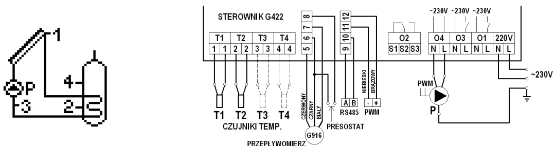
Schemat 1. Schemat ideowy oraz elektryczny instalacji nr 1.
