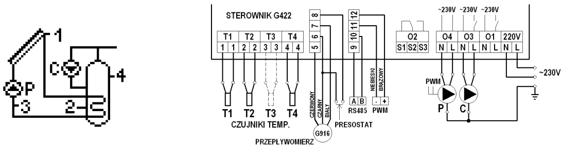
Schemat 2. Schemat ideowy oraz elektryczny instalacji nr 2.
