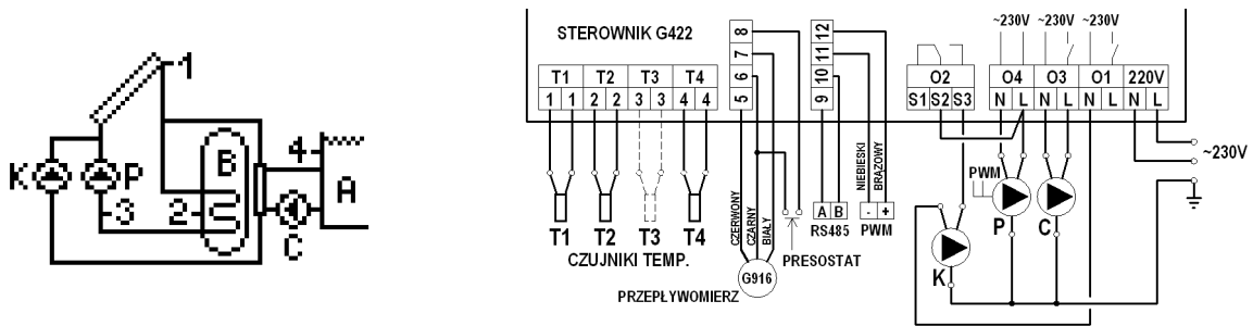
Schemat 10. Schemat ideowy oraz elektryczny instalacji nr 10.
