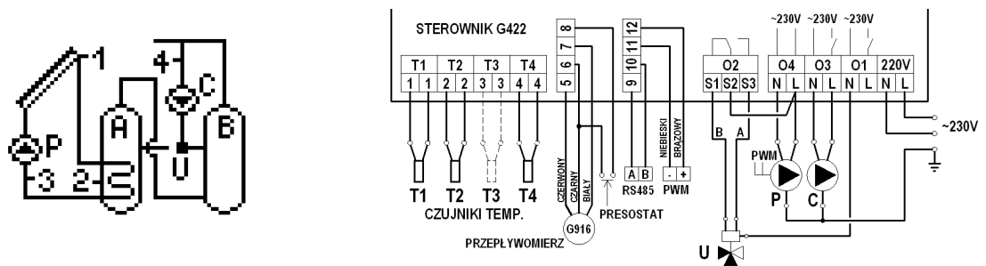
Schemat 8. Schemat ideowy oraz elektryczny instalacji układu nr 8.
