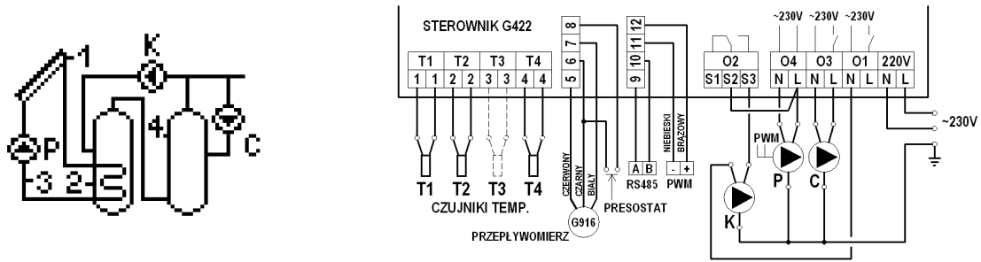
Schemat 7. Schemat ideowy oraz elektryczny instalacji nr 7.
