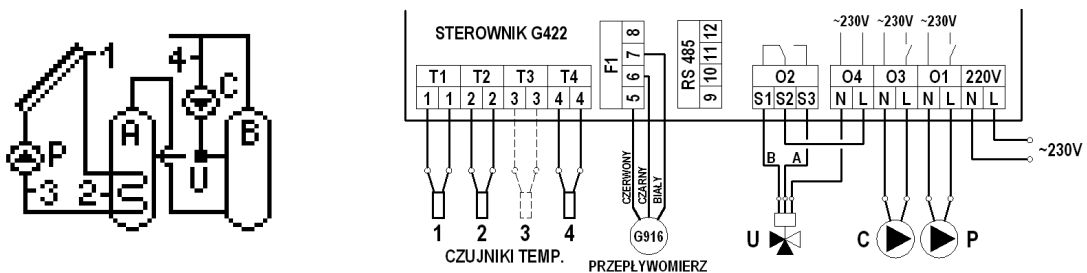
Rys. 10. Schemat ideowy oraz elektryczny instalacji układu nr 8.
