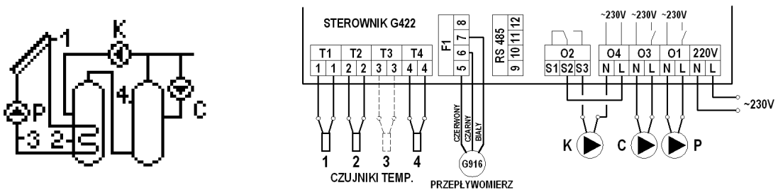
Rys. 9. Schemat ideowy oraz elektryczny instalacji nr 7.
