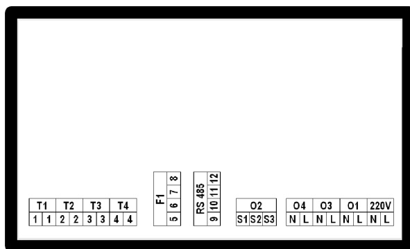
Rys. 1. Oznaczenie wejść i wyjść sterownika.
