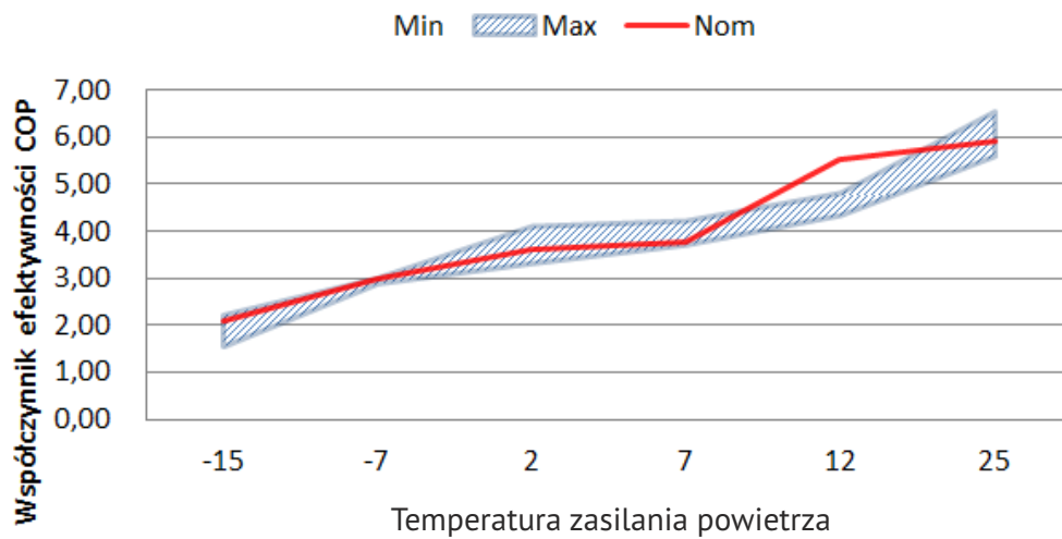
COP dla temperatury powrotu z instalacji 30°C
