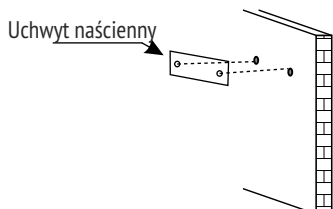
A. Zaznacz otwory w ścianie. Wypoziomuj je.
