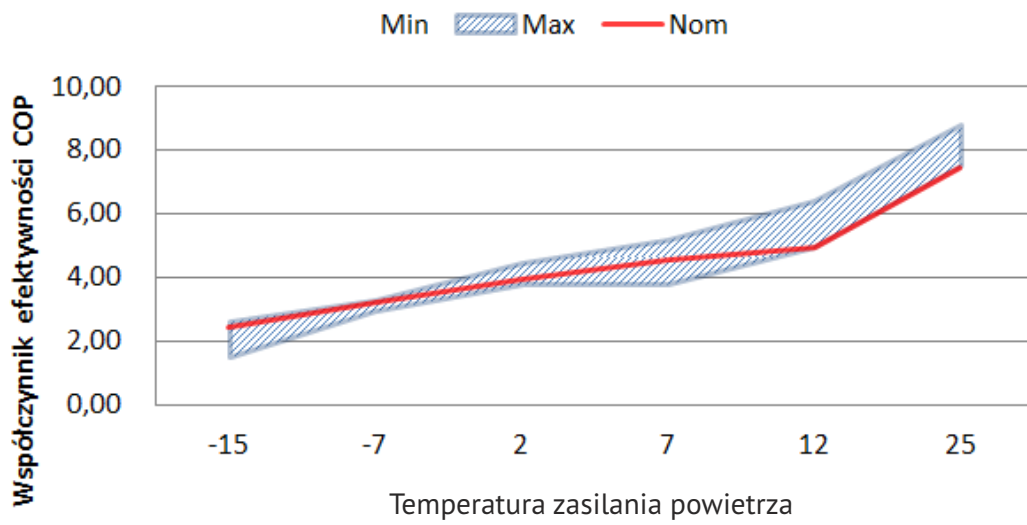
COP dla temperatury powrotu z instalacji 20°C
