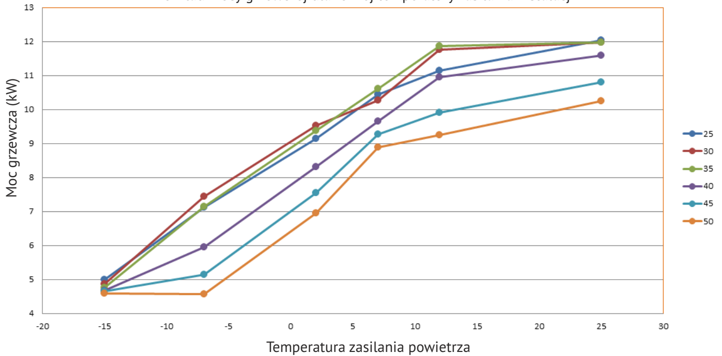
Rozkład mocy grzewczej dla różnej temperatury zasilania instalacji
