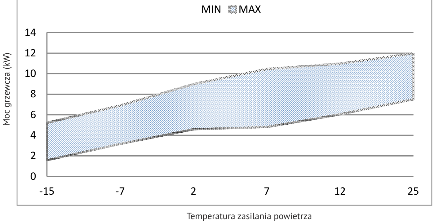
Rozkład mocy grzewczej dla temperatury powrotu z instalacji 20°C
