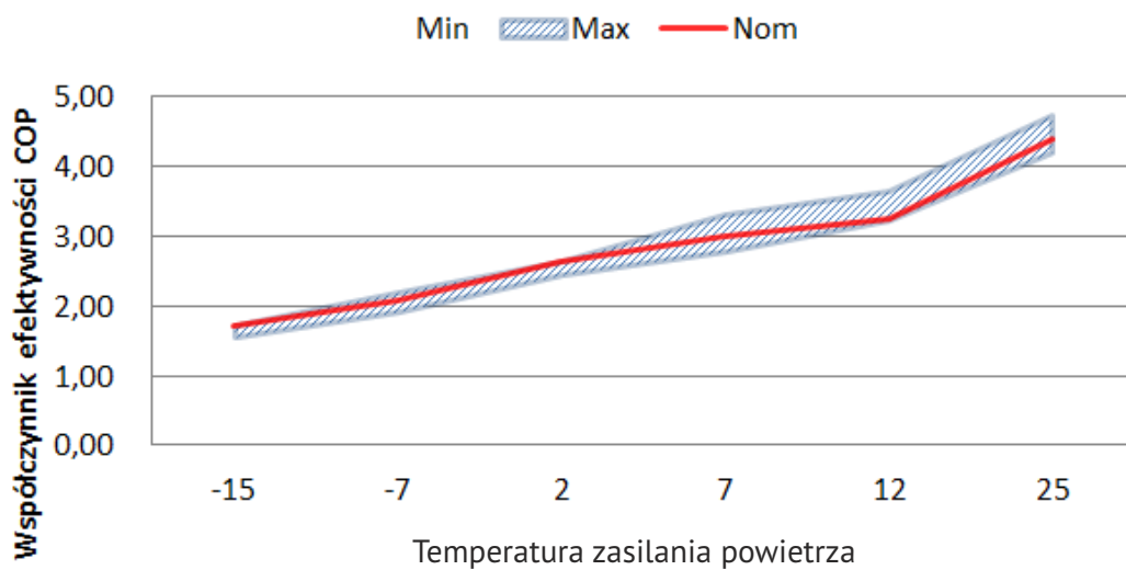
COP dla temperatury powrotu z instalacji 40°C
